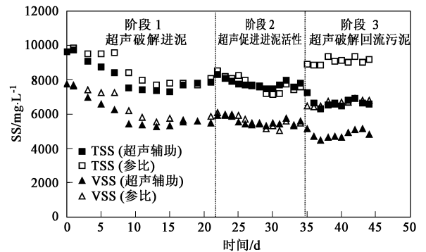
图 3 超声处理辅助污泥好氧消化的效果
