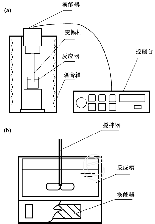
图 1 超声处理实验装置示意
